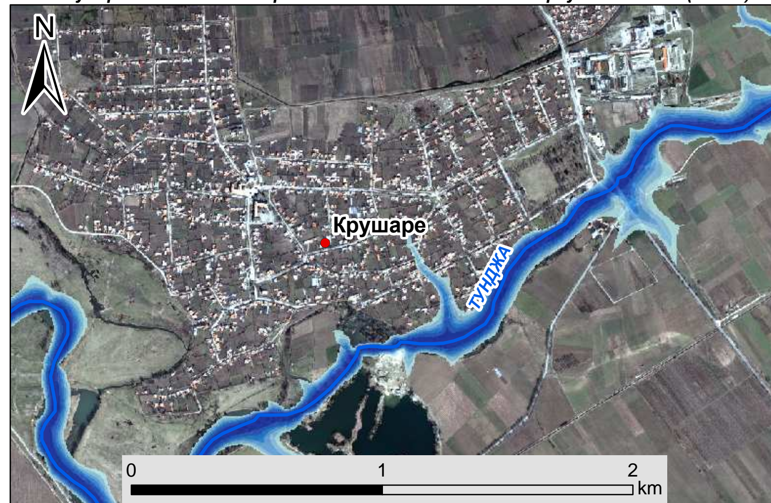
Симулирано наводнение при височина на вълната 5м върху QUICKBIRD (0.70 м)
