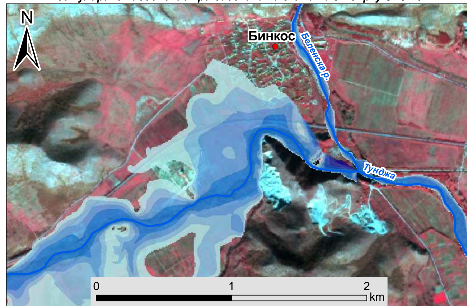
Симулирано наводнение при височина на вълната 5м върху SPOT 5
